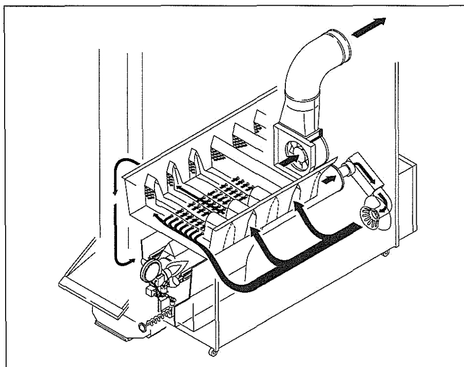
【内部構造図】
