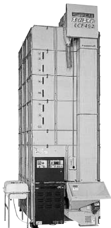
Photo:ECF402-SND
